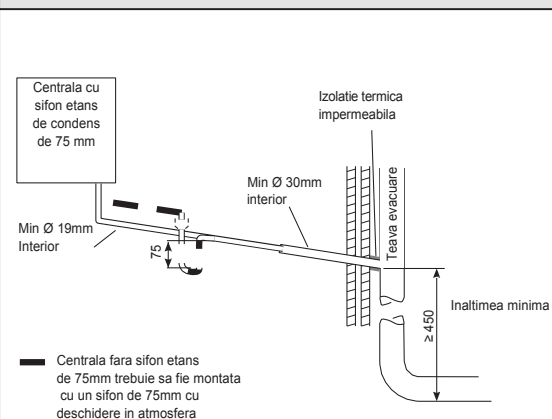
Figura 4 – Conectarea la un sistem de evacuare exterior
