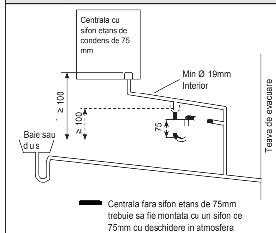
Figura 2 – Conectarea sistemului de evacuare al condensului la teava de descarcare internă a unui alt sifon (baie, dus, chiuvetă, etc.)
