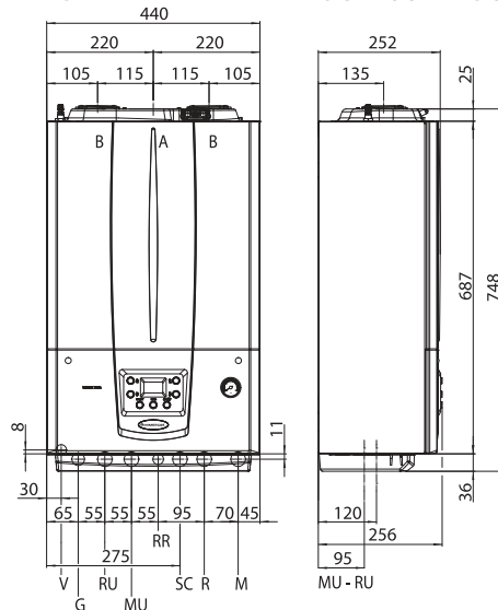
VICTRIX TERA 24 PLUS - 35 PLUS
