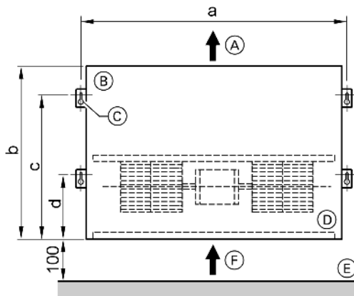
Fixare pe perete (vedere din față)
