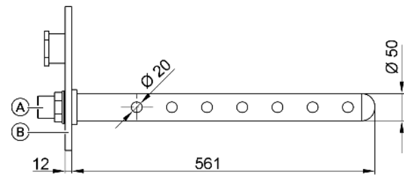
Lance de încărcare
