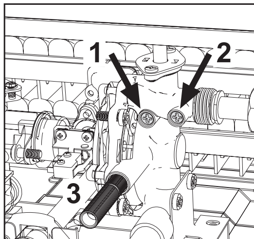
fig. 9 - Șuruburi de reglare a debitului de apă
