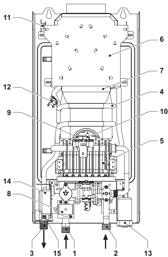
fig. 22 - Vedere generală ZEFIRO ECO 6
