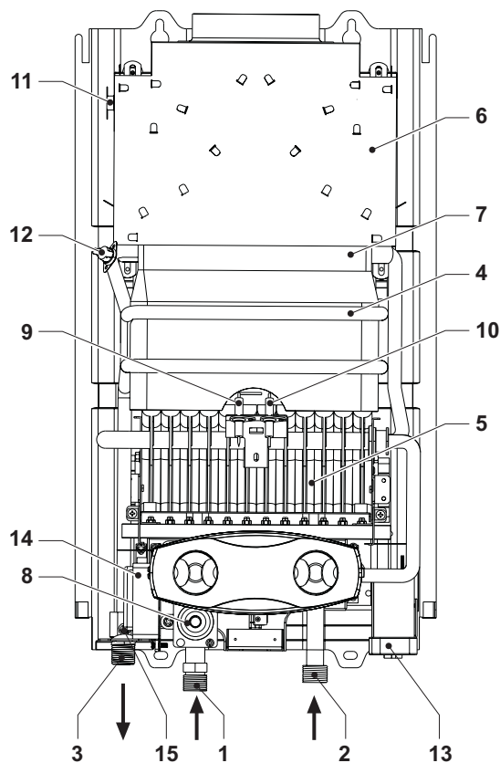
fig. 23 - Vedere generală ZEFIRO ECO 11
