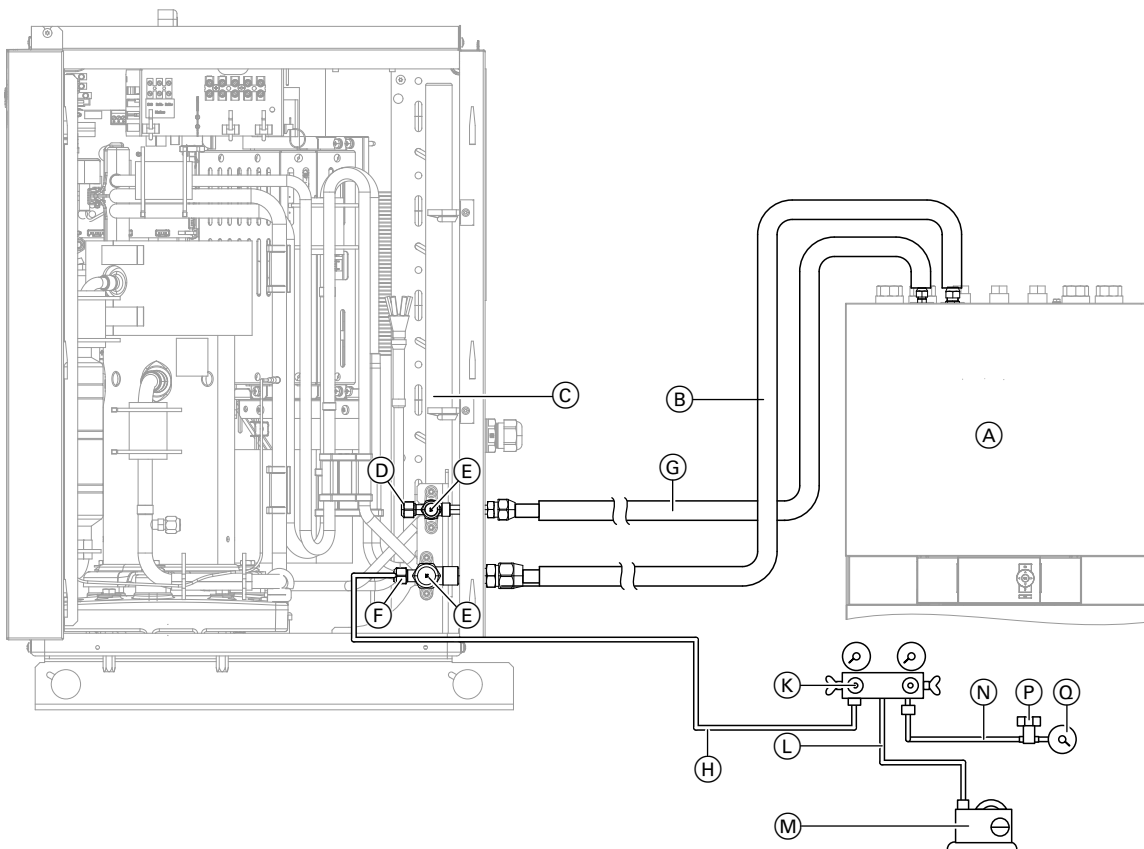
Fig. 61 Exemplu tip AWBT-M-E-AC 222.C06
