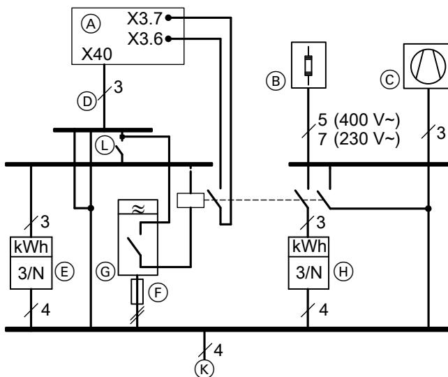
Fig. 56 Reprezentare fără siguranțe și fără întrerupător de protecție FI
