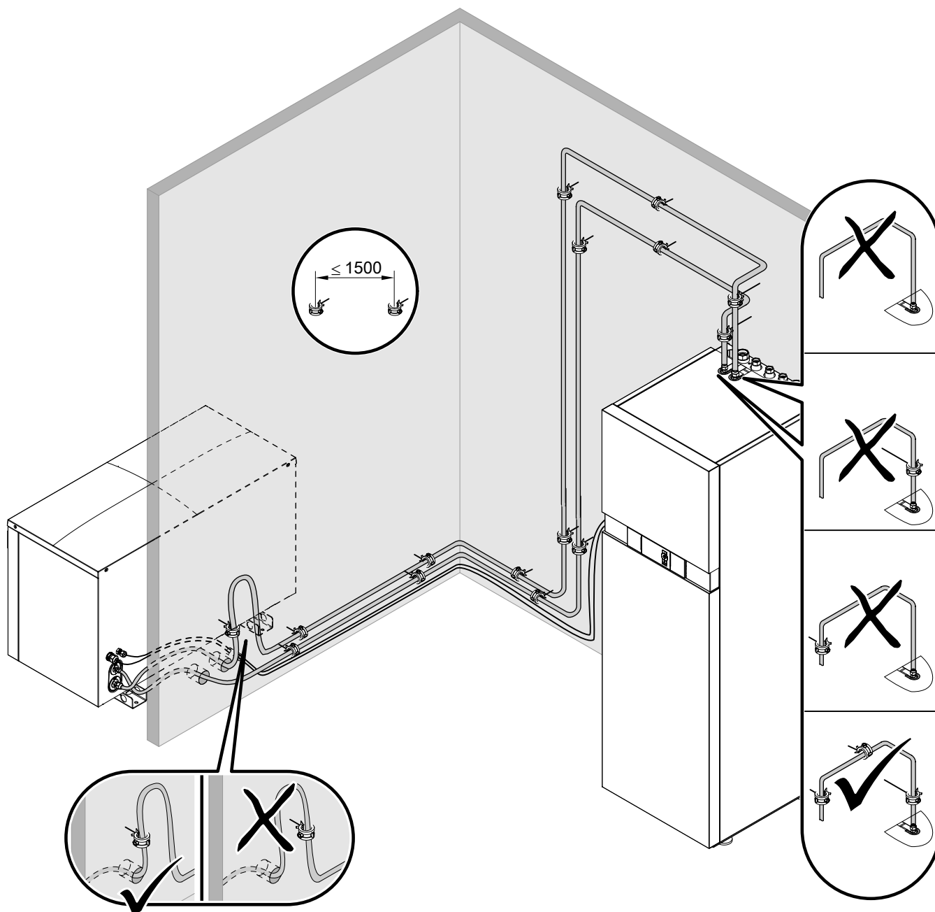
Fig. 26 Cot pentru compensarea vibrațiilor în interiorul clădirii
