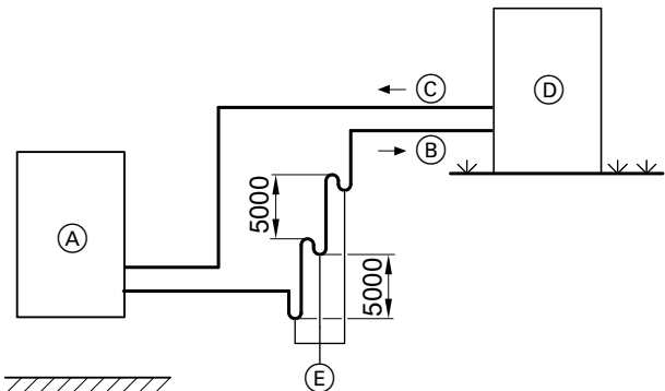
Fig. 23 Exemplu de regim de răcire: Cu coturi de ulei
