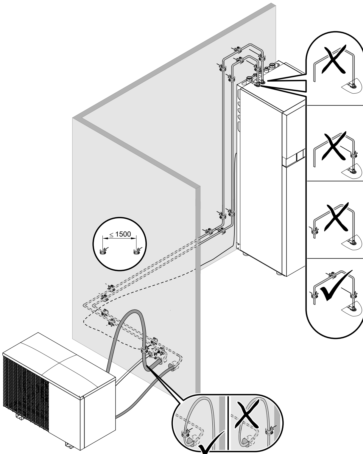
Fig. 25 Cot pentru compensarea vibrațiilor în afara clădirii
