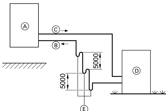
Fig. 22 Exemplu de regim de încălzire: Cu coturi de ulei
